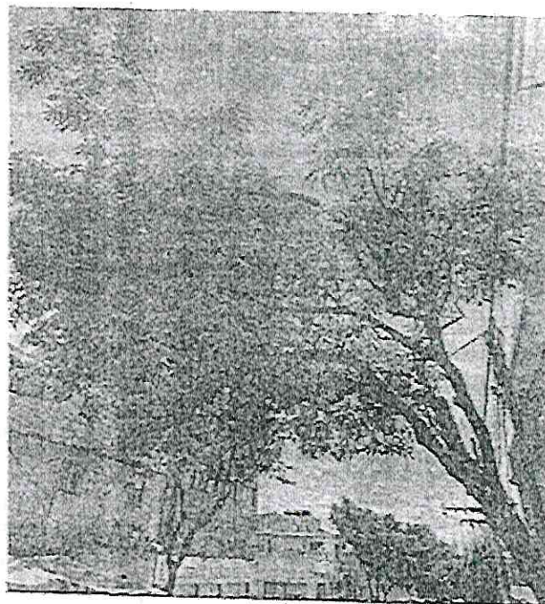
Árbol 1
