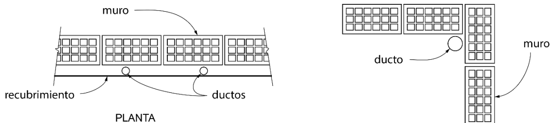
Figura 9.2.2 Ejemplos de ductos fuera del muro
