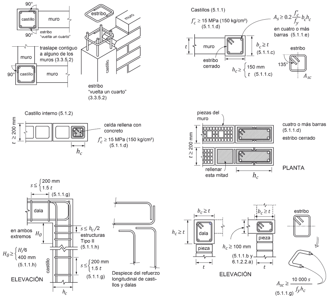
Figura 5.1.2 Castillos y dalas
